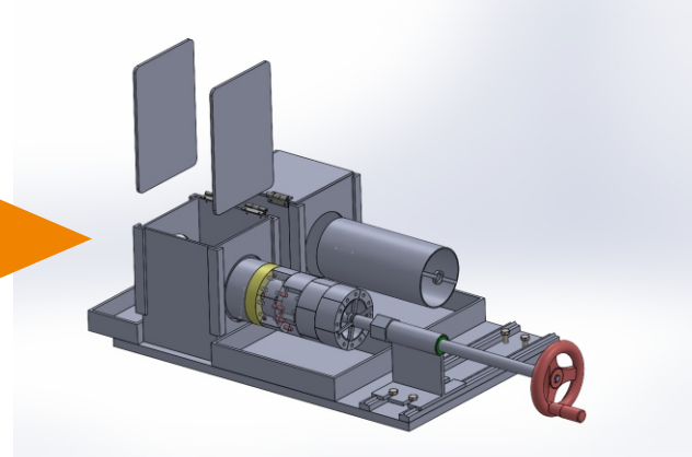
構想図
