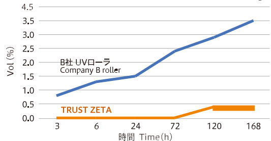
環境対応型洗浄液に対する耐性 Resistance properties against Environmental responsiveness solvent
