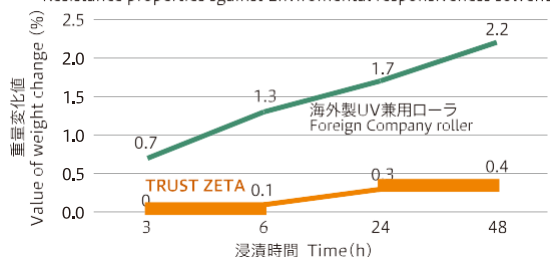
環境対応型洗浄液に対する耐性 Resistance properties against Environmental responsiveness solvent
